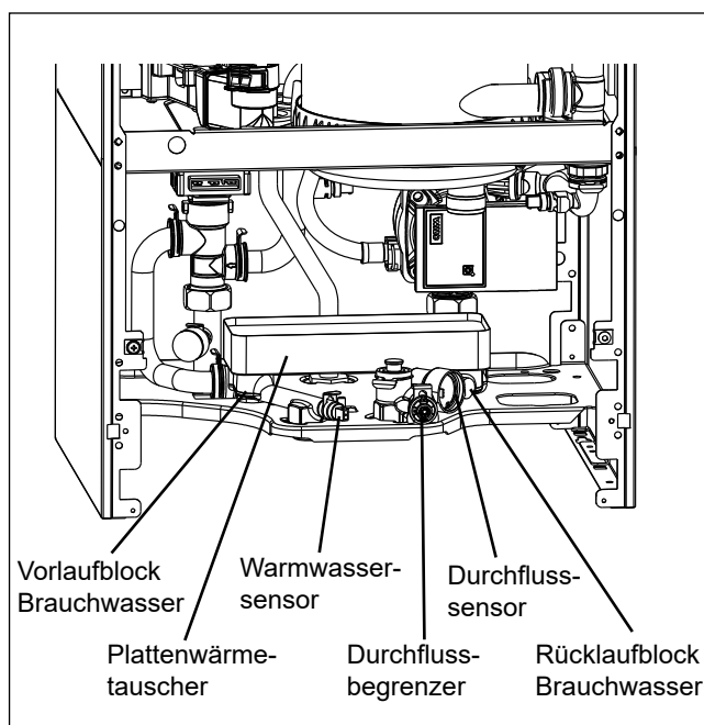
Bild: Verrohrung Kombigerät
