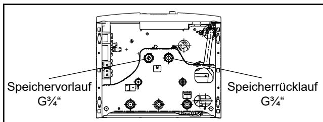
Bild: Speichervorlauf- / rücklauf Anschluss
