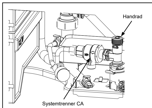
Bild: Befülleinrichtung als Nachrüstungsset im Gerät integrierbar
