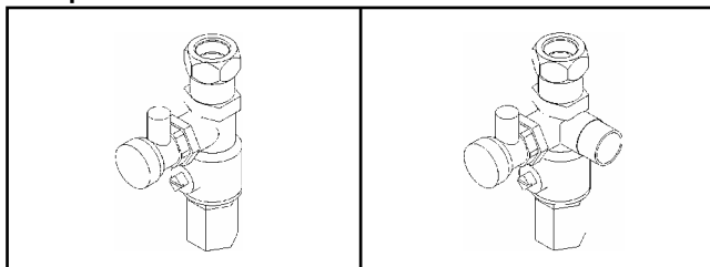
Bild: Durchgangswartungshahn, mit KFE-Hahn (Zubehör)
