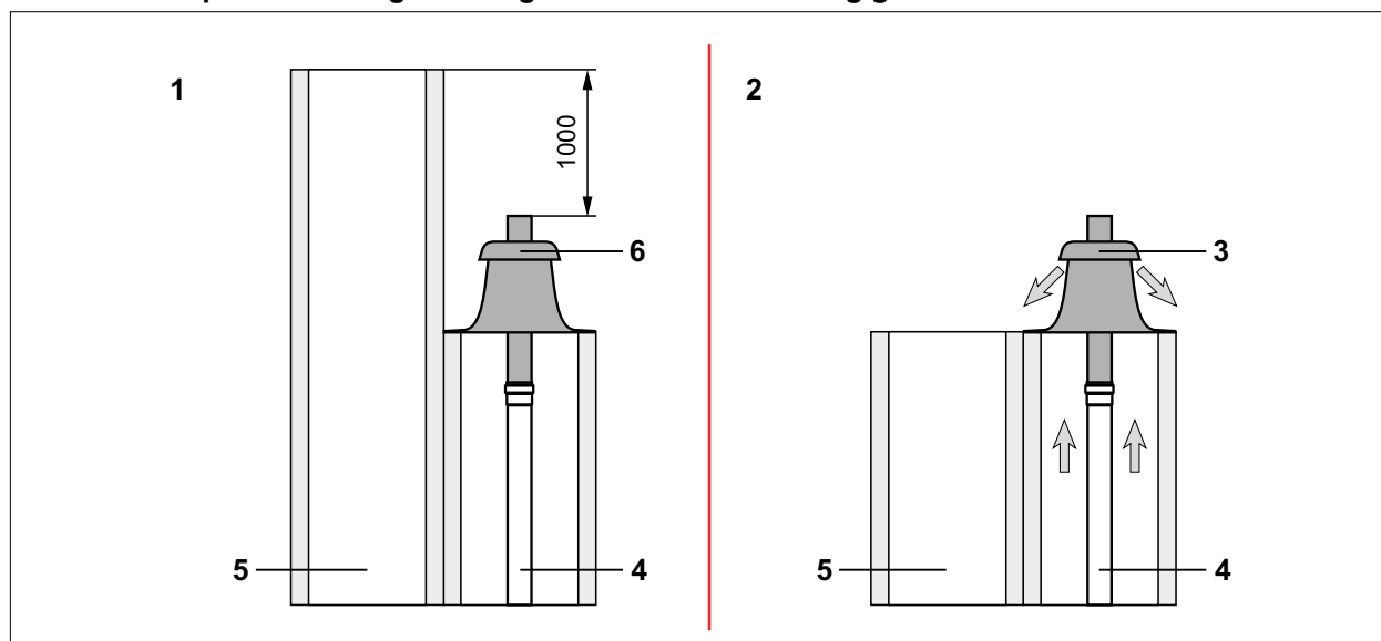
Abb. 4.6 Zweizügiger Schornstein
