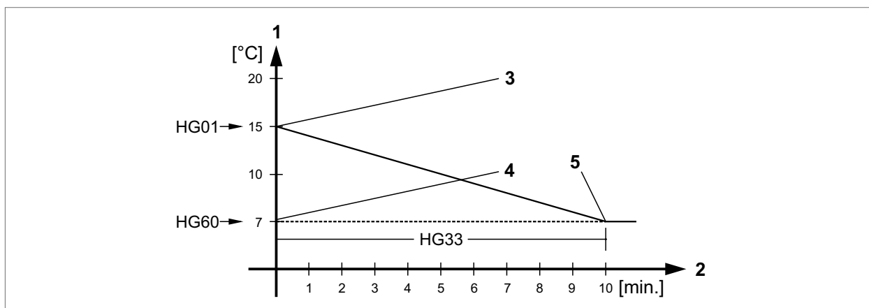
Abb. 7.1 Brennerhysterese
