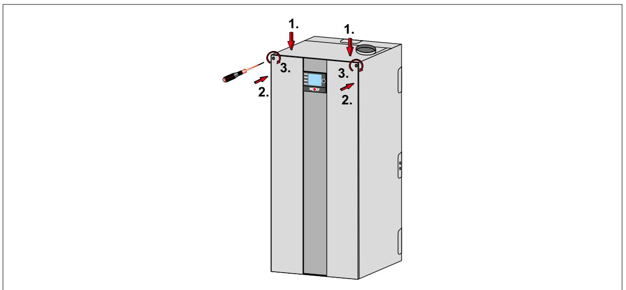
Abb. 5.3 Verkleidung montieren
