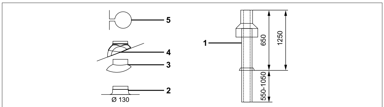
Abb. 5.16 Dachdurchführung [mm]
