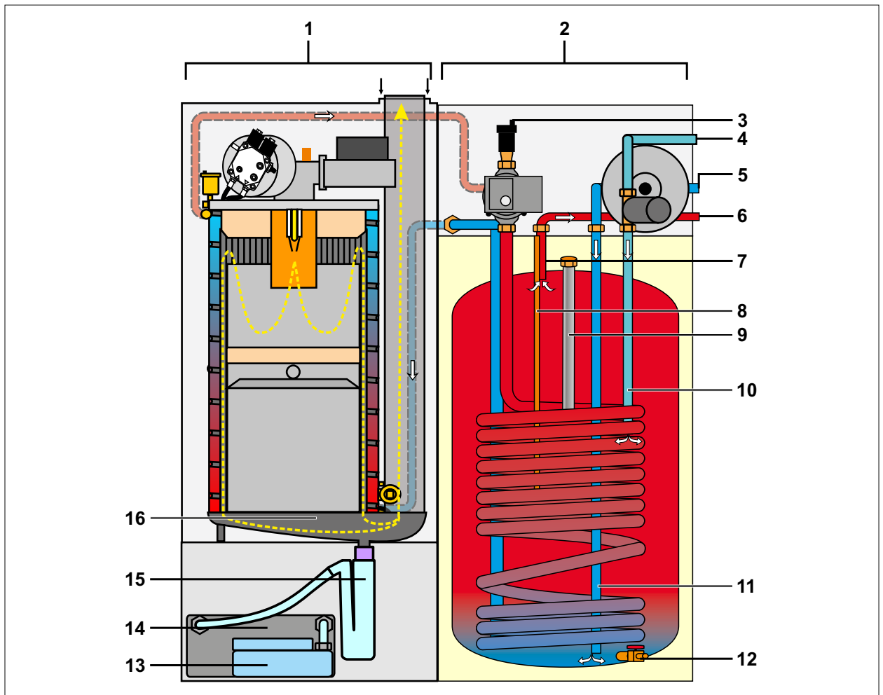
Abb. 3.2 Aufbauschema Ölheizwertkessel COB-2 mit TR
