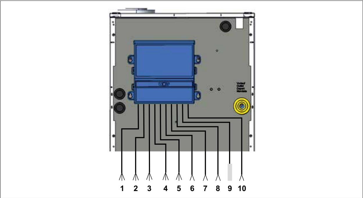
Abb. 5.23 Elektroanschluss Reglungskasten
