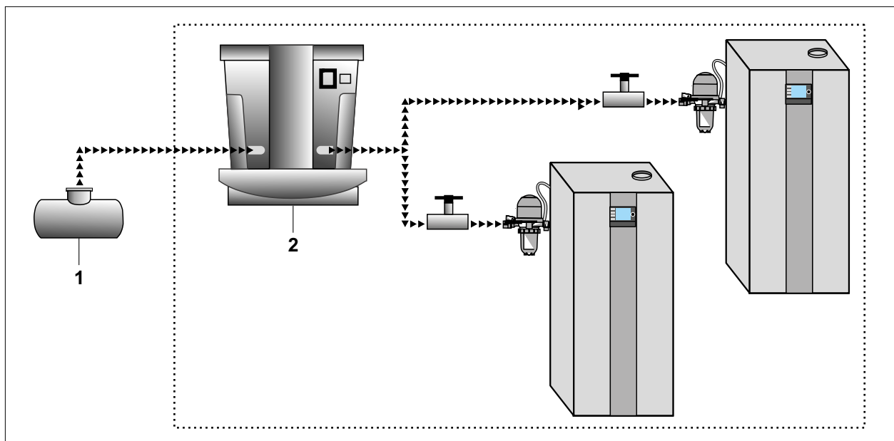
Abb. 4.8 Brennstoffversorgung
