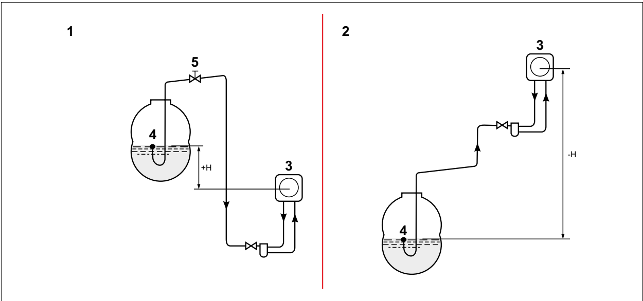
Abb. 4.3 Schwimmende Absaugung
